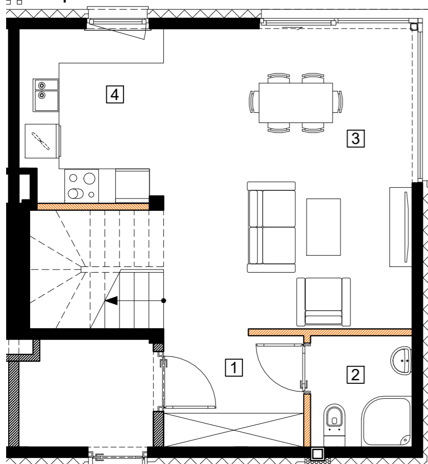
Rzut parteru
